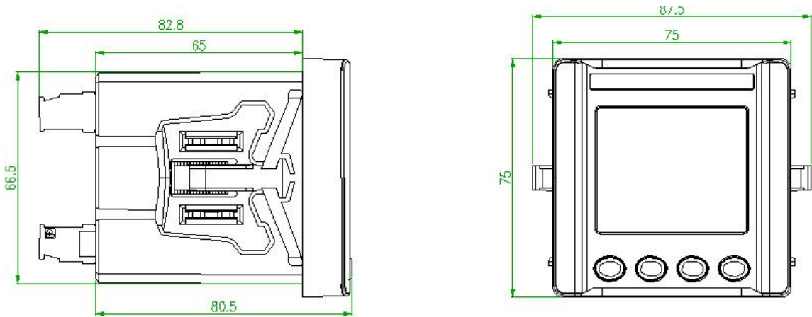
图 2 APM510 尺寸图
