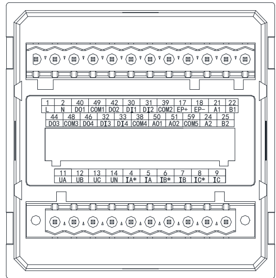
图 8 APM510 扩展 K/2M/2C 接线图
